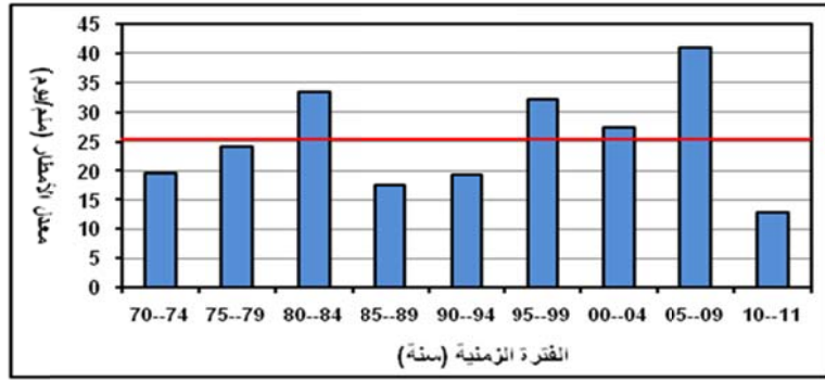
الشكل ٨ : معدلات الأمطار اليومية القصوى للفترة ١٩٧٠ - ٢٠١١ م بمحطة حريملاء
