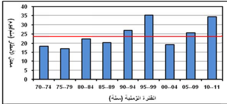
الشكل ٤ : معدلات الأمطار اليومية القصوى للفترة ١٩٧٠ - ٢٠١١ م بمحطة شقراء
