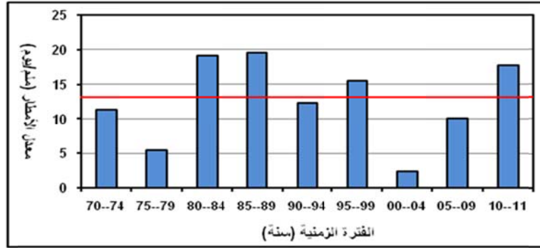
الشكل ١١ : معدلات الأمطار اليومية القصوى للفترة ١٩٧٠ - ٢٠١١ م بمحطة الخرج
