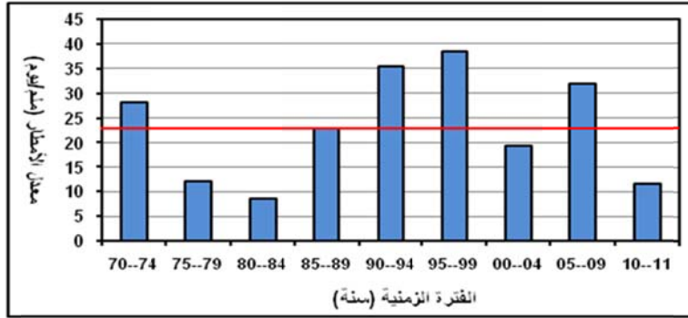
الشكل ٩ : معدلات الأمطار اليومية القصوى للفترة ١٩٧٠ - ٢٠١١ م بمحطة الجمعة
