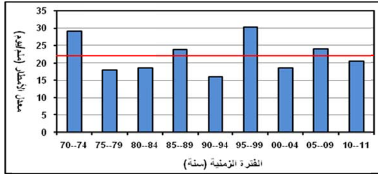
الشكل ٥ : معدلات الأمطار اليومية القصوى للفترة ١٩٧٠ - ٢٠١١ م بمحطة سدوس
